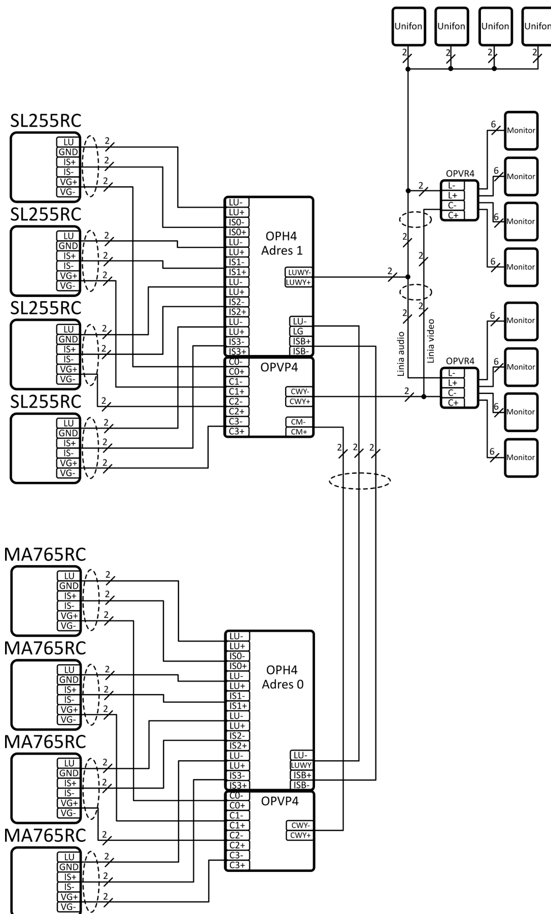
Ilustracja 5: Praca paneli SL255RC i MA765RC w przykładowym systemie Master-Slave wideo
